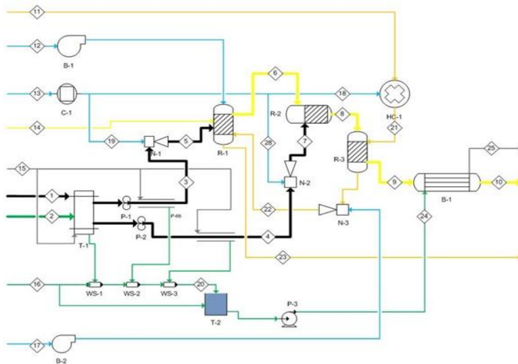
Gambar 3.1 Rancangan PFD untuk Gasifikasi Reforming Ter
